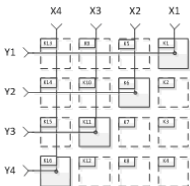
Поле допустимых точек коммутации
